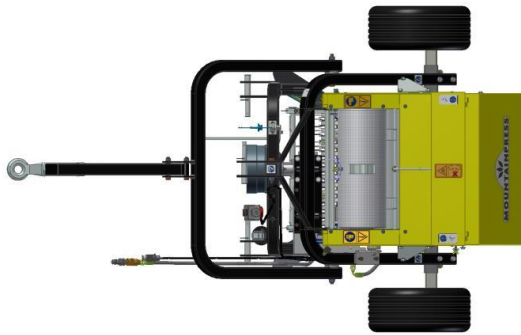
Abb. 6 Mittige Deichsel
