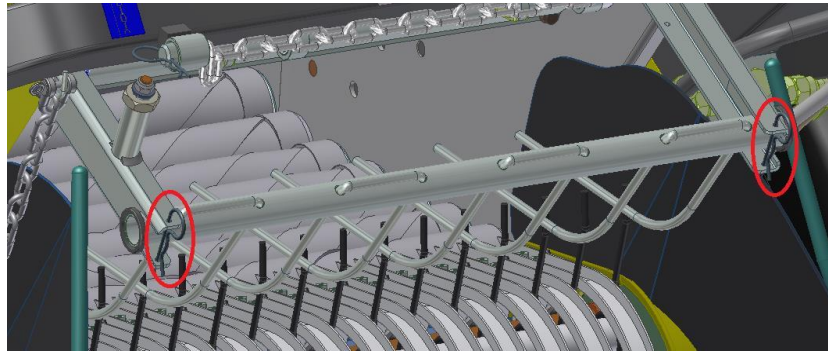
Abb. 16 Position der elastischen Splints des Förderrechen
