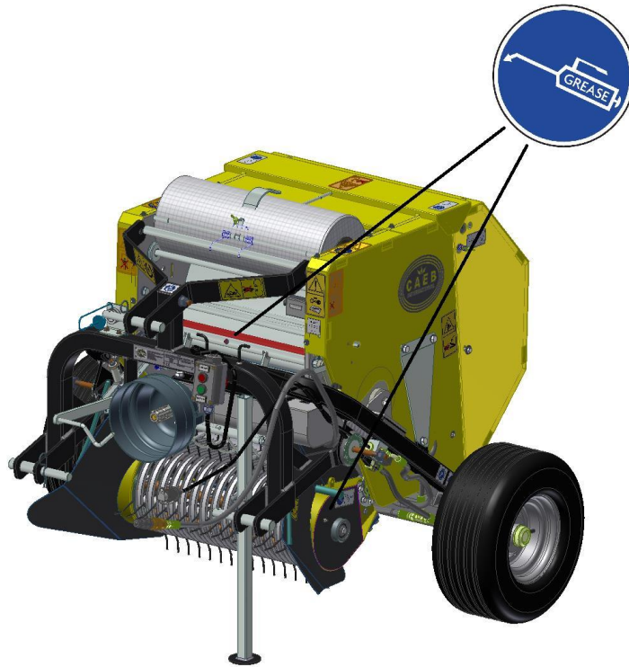
Abb. 228 Einfettungspunkte
