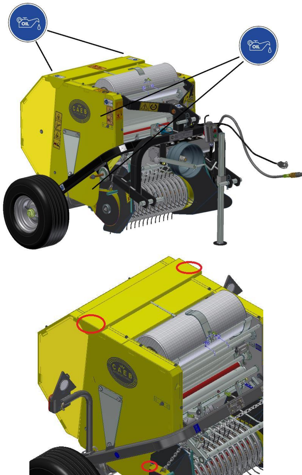
Abb. 39 Schmierungspunkte
