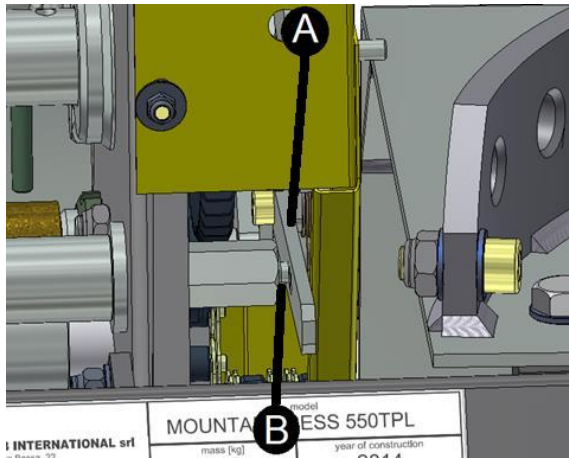
Abb. 101 Einstellhebel A, Fixierzapfen B
