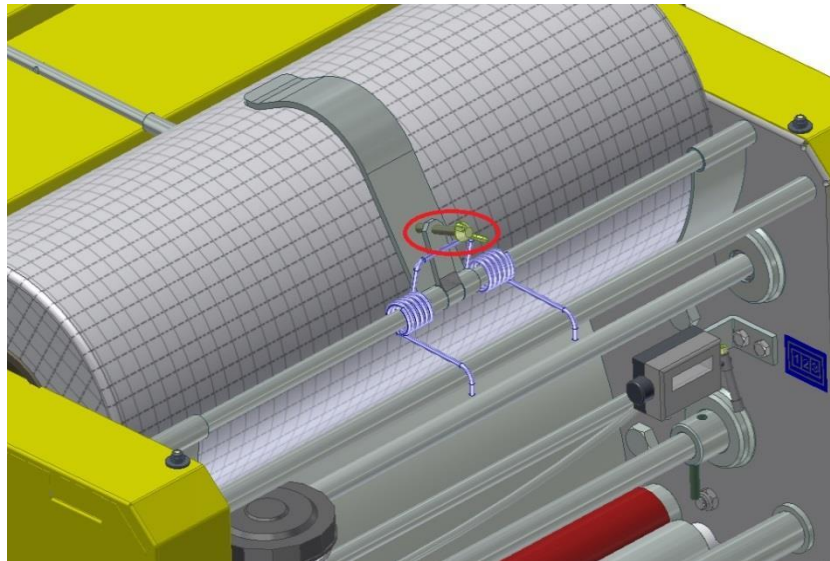
Abb. 140 Einstellung der Netzbremse
