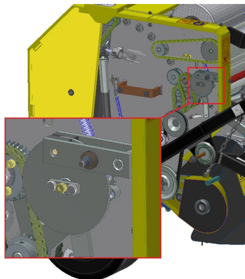
Abb. 184 Freno legata Bindungsbremse
