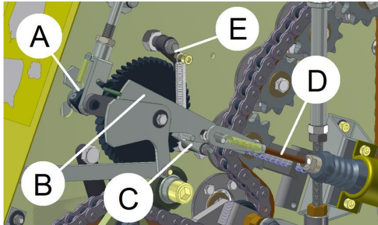
Abb. 231 Reinigung des Bindungsmechanismus
