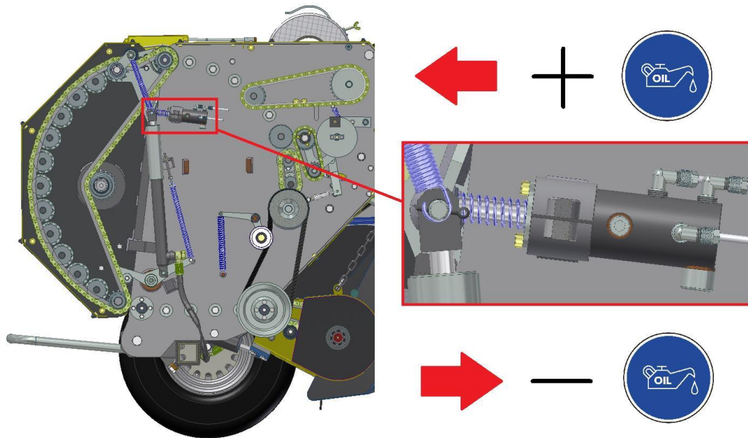
Abb. 29 Einstellung der Schmierpumpe
