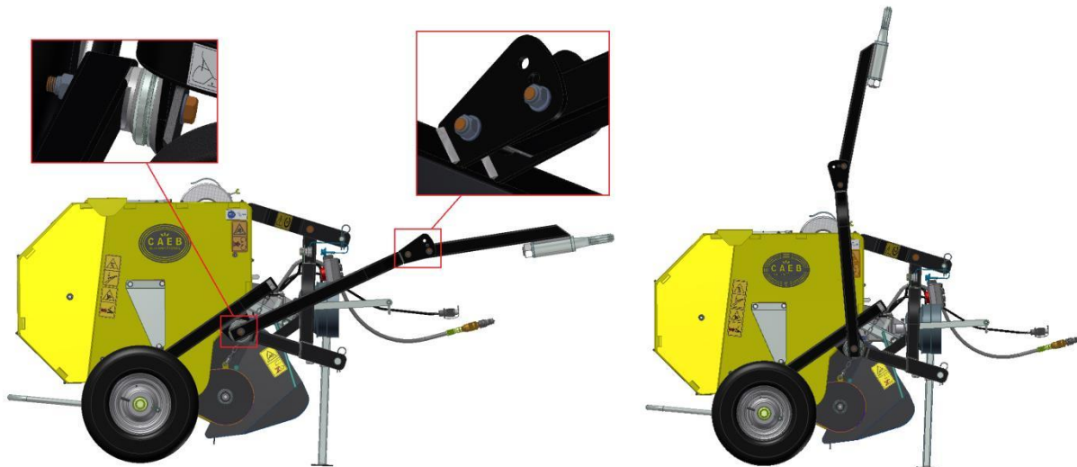
Abb. 25 Anschlusspunkte des Abschleppsatzes
