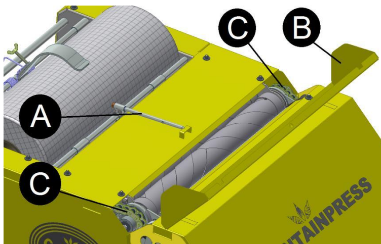
Abb. 217 Schmierungspunkte der Rollenantriebsketten
