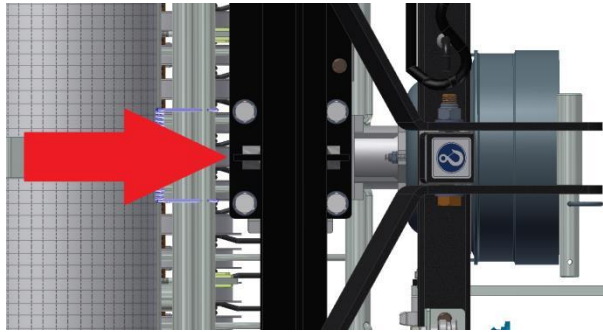
Abb. 40 Einfüllstopfen für Winkeltrieböl
