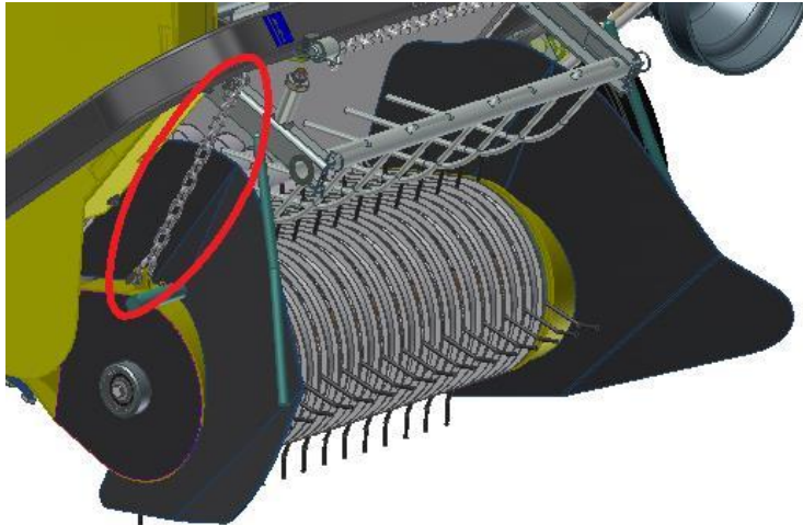
Abb. 19 Einstellkette des Greifers
