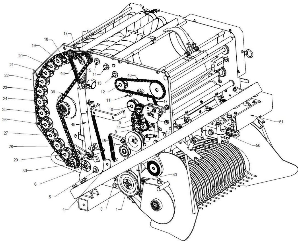
Abb. 286 Ziffern für die Feststellung der Übergruppen an der rechten Seite (Fahrriichtung)
