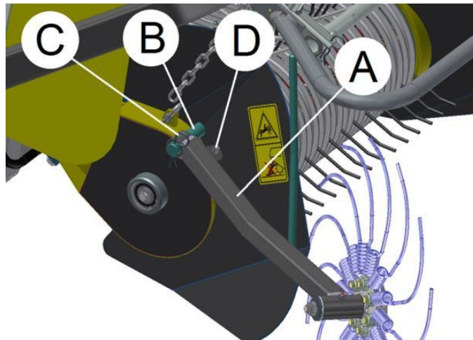
Abb. 134 Montage der Schwadenräder
