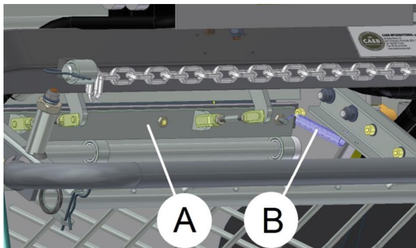
Abb. 151 Rückstellfedern des Kontermessers
