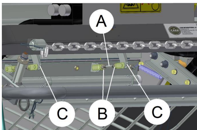
Abb. 206 Einstellung der Kontermesserscheibe
