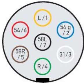
Abb. 297 Anordnung der Steckdosenkontakte Typ 12N
