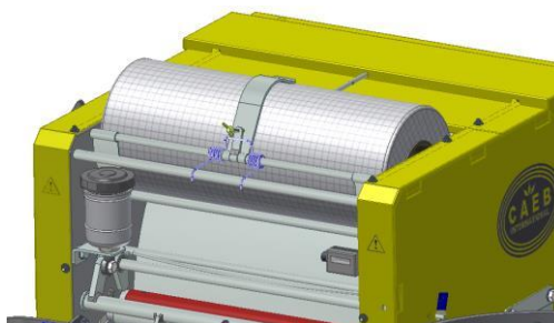
Abb. 4 Schmierung
