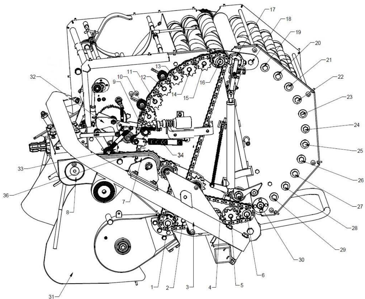
Abb. 275 Ziffern für die Feststellung der Übergruppen an der linken Seite (Fahrriktion)
