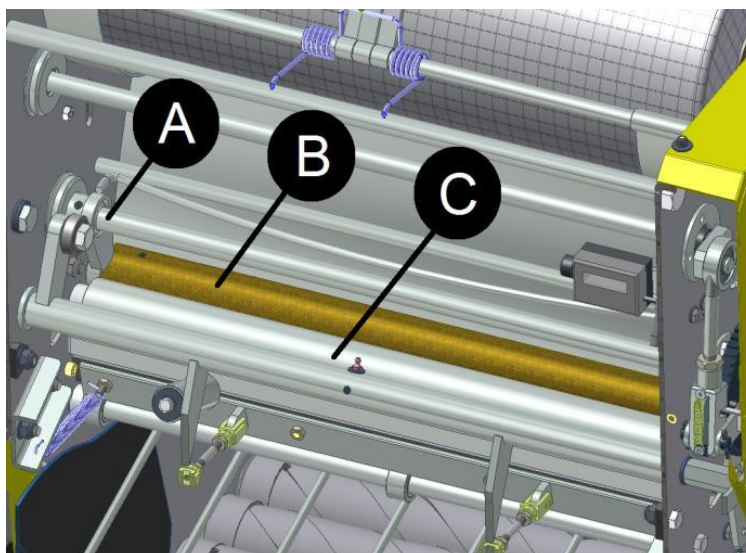
Abb. 195 Antriebsrollen in den Leerlauf versetzen
